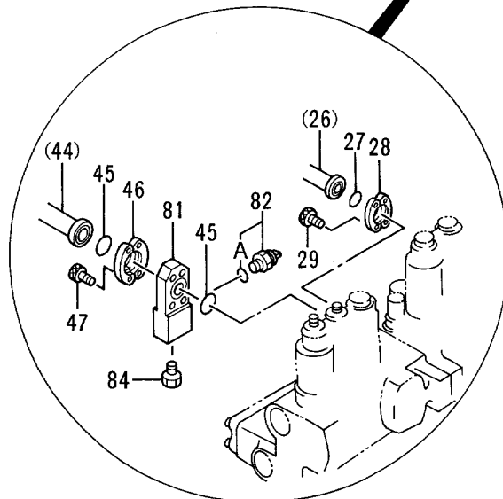
バルブ ; コントロール VALVE ; CONTROL
