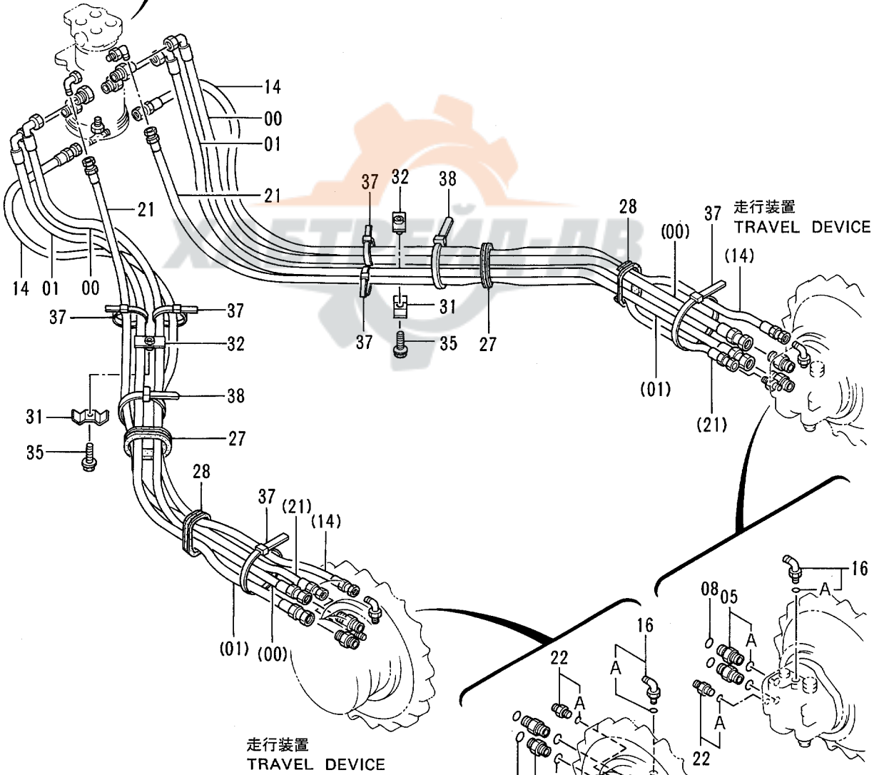
センタージョイント CENTER JOINT
