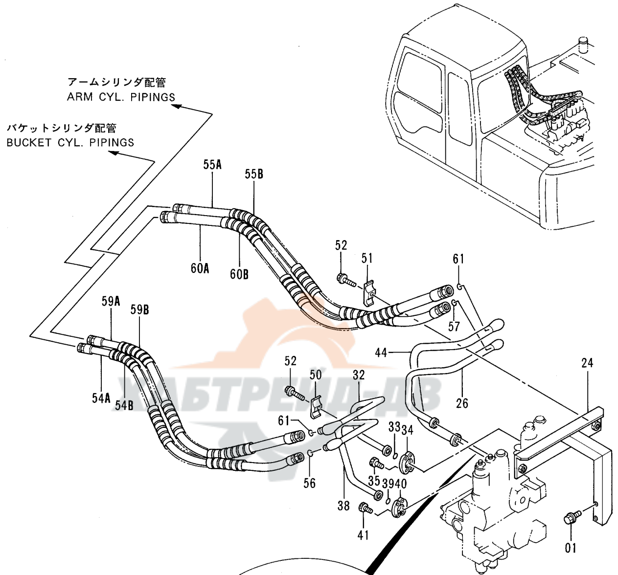
バルブ ; コントロール VALVE ; CONTROL
