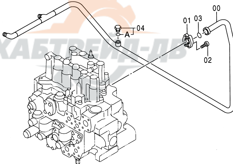
コントロールバルブ CONTROL VALVE
