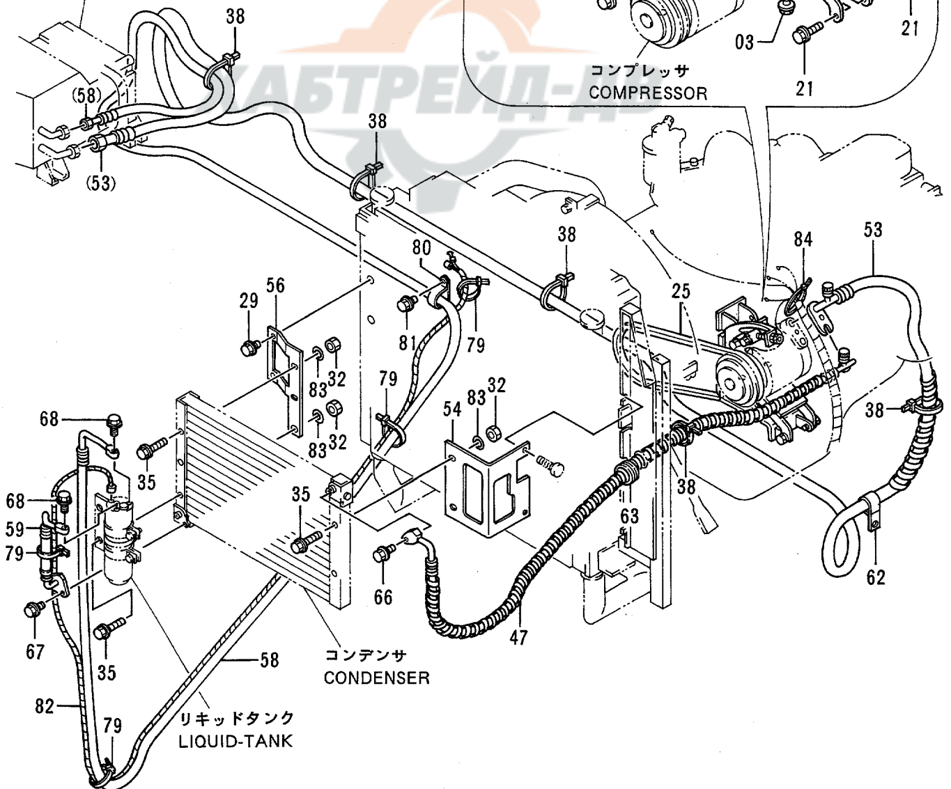
エアコンユニット AIR-CON. UNIT
